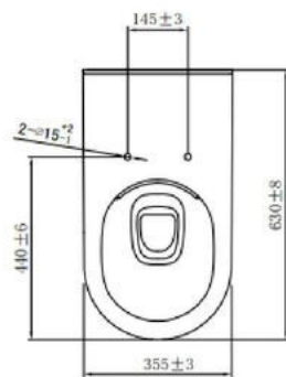
TOP VIES
